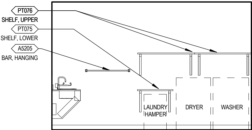
Elevation 2
