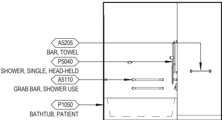
Elevation 6
