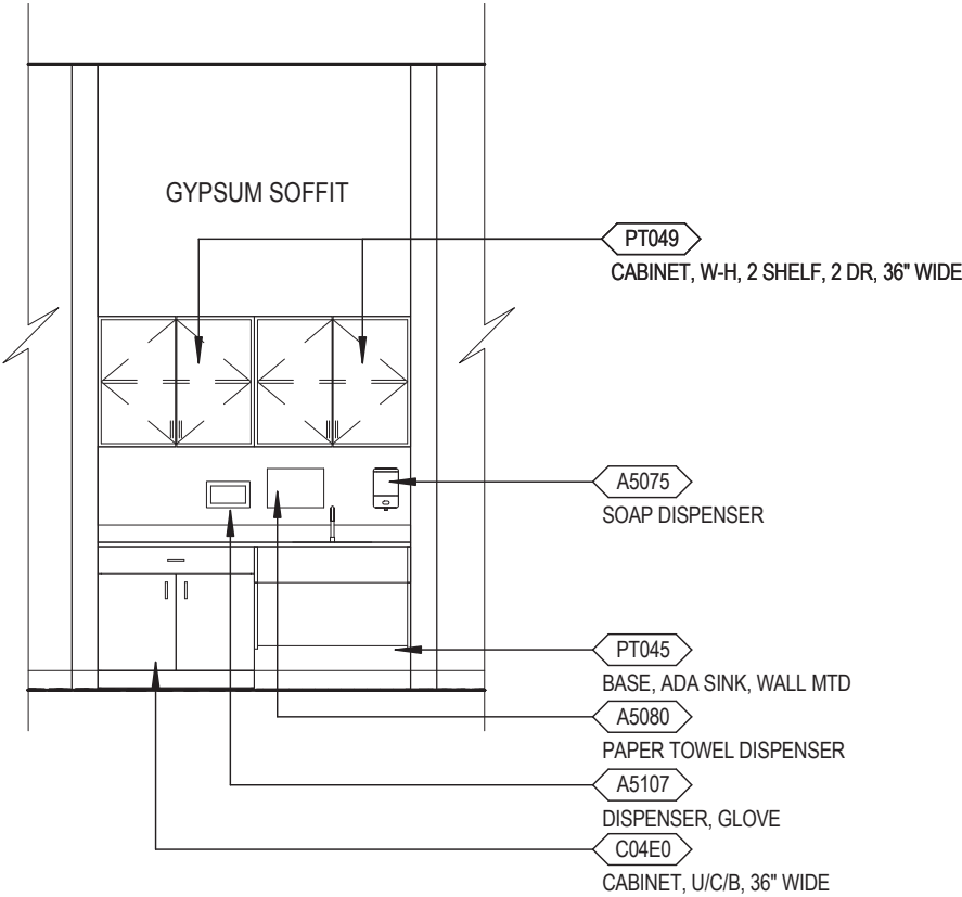
Elevation 2
