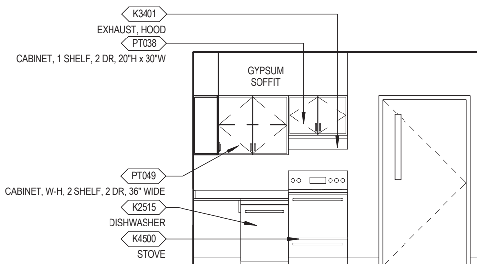
Elevation 1
