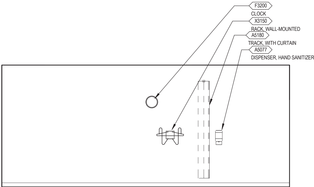
Elevation 1
