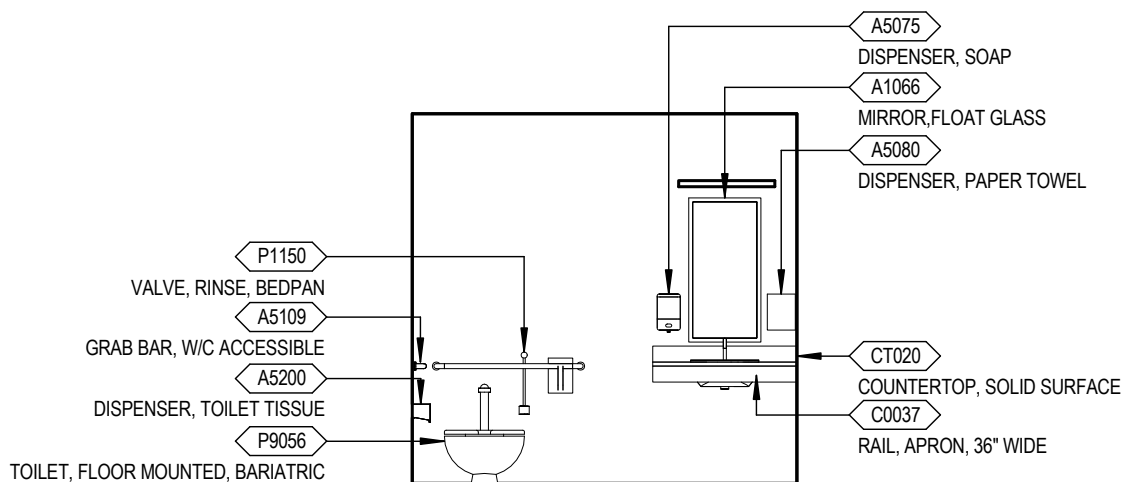
Elevation 4
