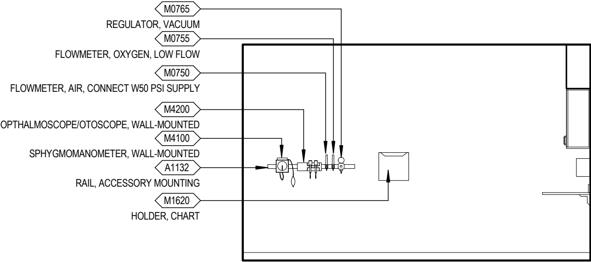
Elevation 1
