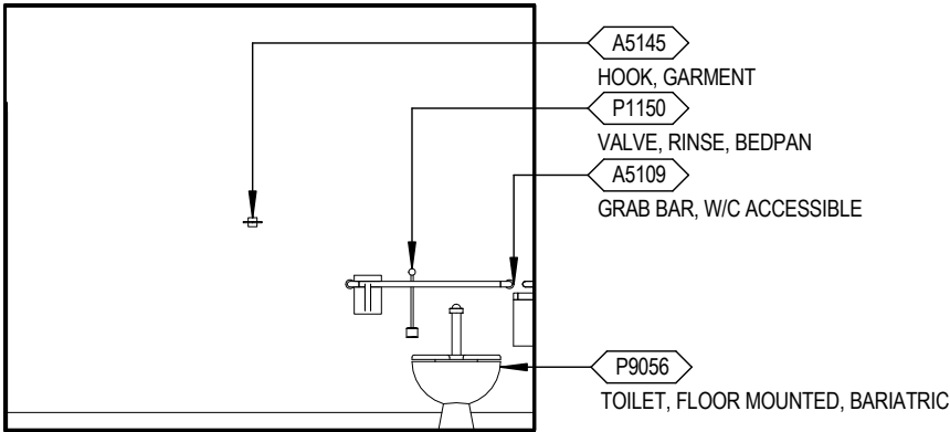
Elevation 2
