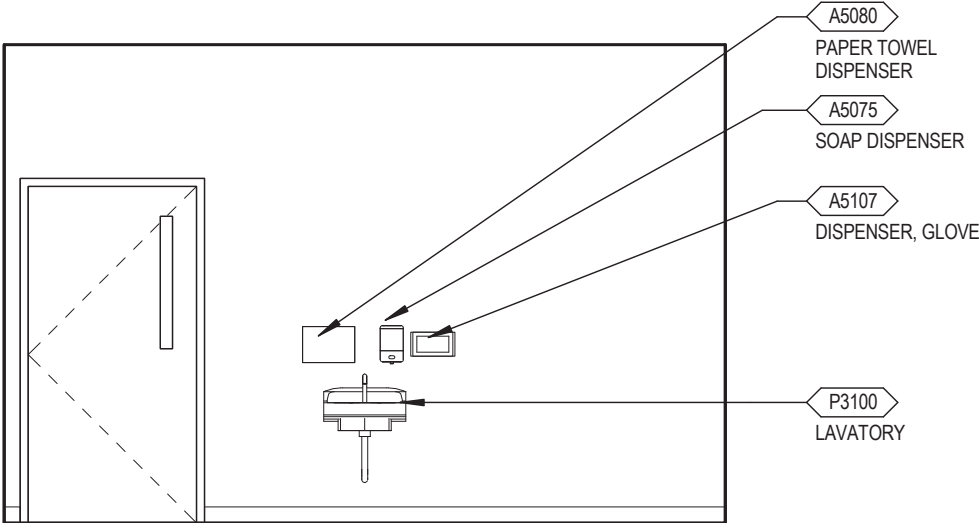
Elevation 2
