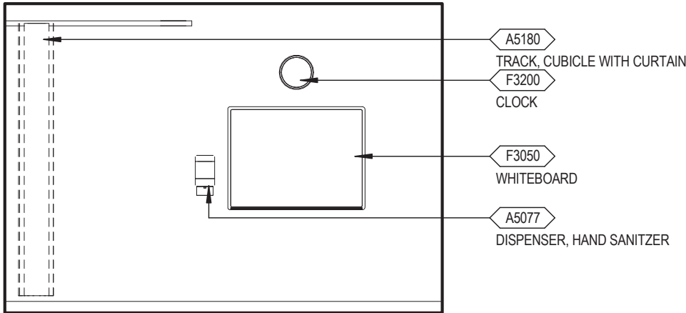
Elevation 4
