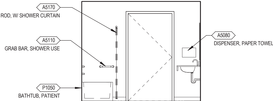
Elevation 4
