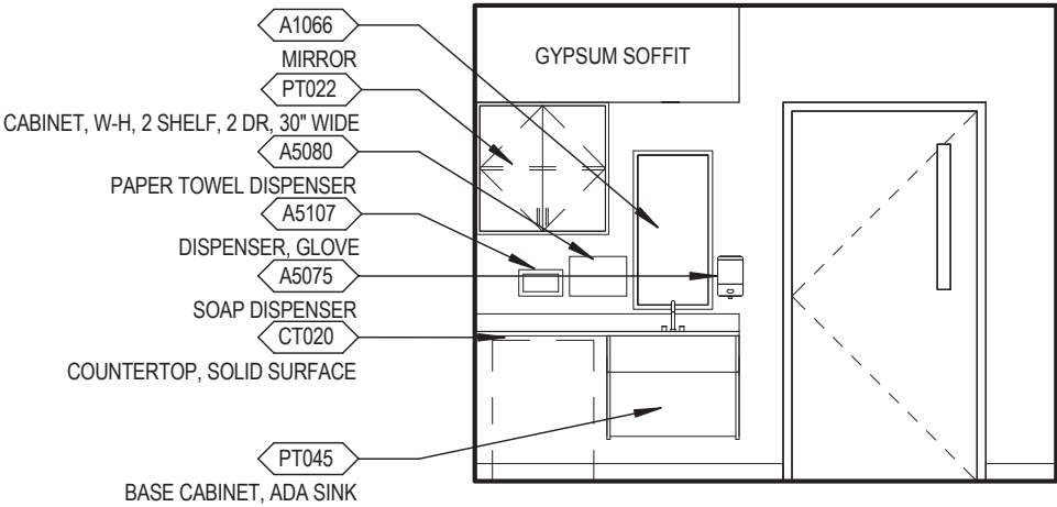
Elevation 3
