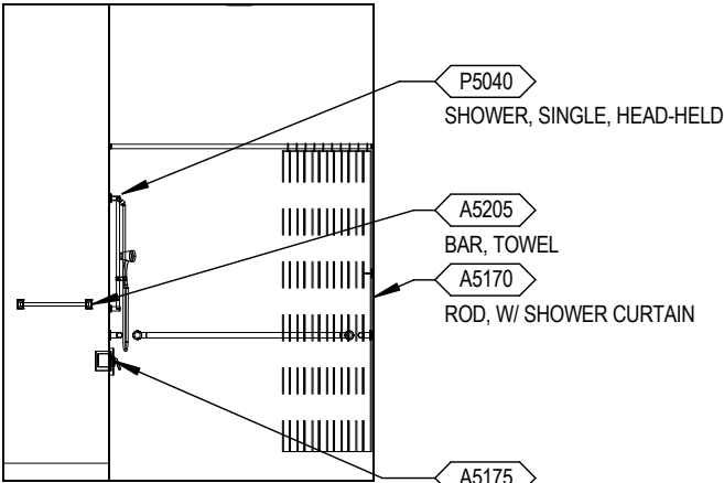
Elevation 7
