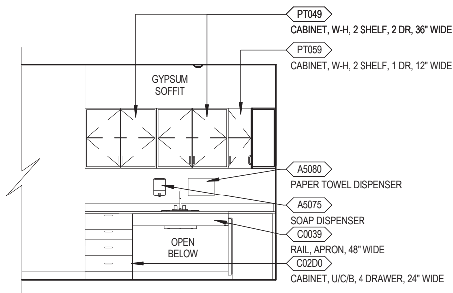
Elevation 2
