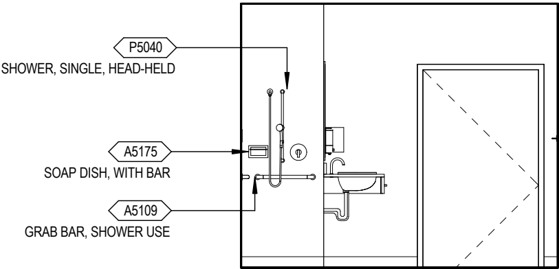
Elevation 1
