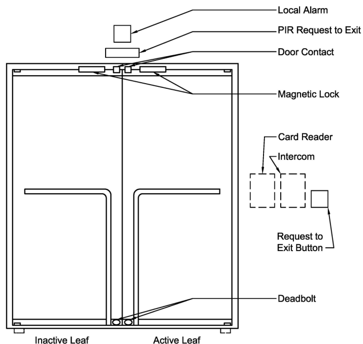
Door Type D - Frameless Pair of Doors
