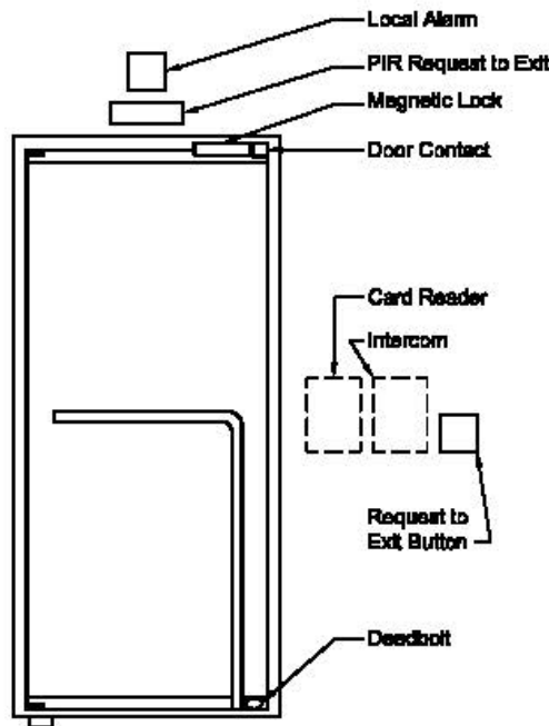
Door Type B - Frameless Single Door
